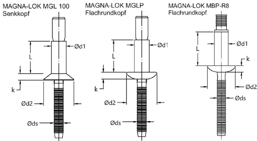
Abbildung A1.1: Hauptabmessungen der Blindniete
