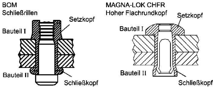
Abbildung A2.2: Blindniete gesetzt
