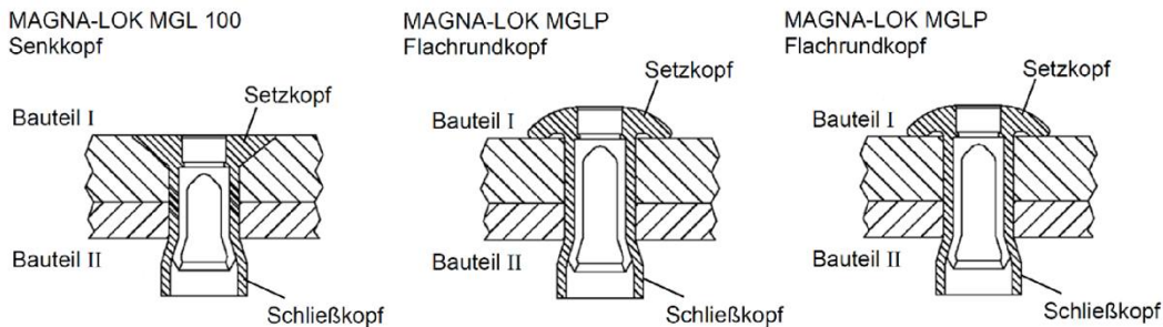
Abbildung A1.2: Blindniete gesetzt
