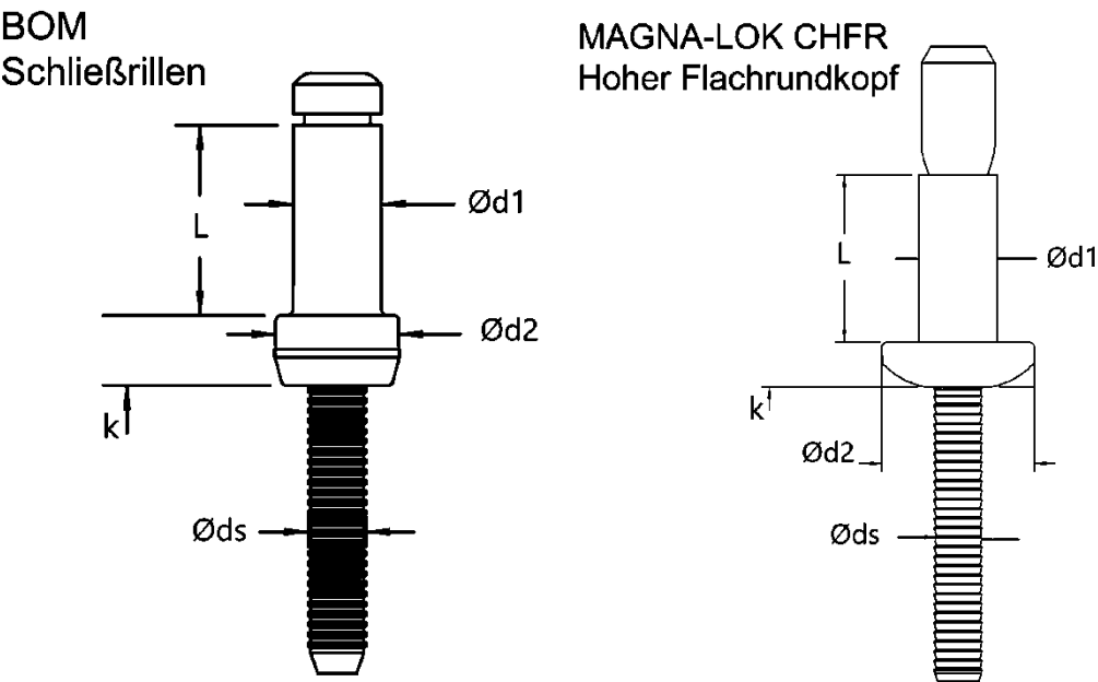
Abbildung A2.1: Hauptabmessungen der Blindniete
